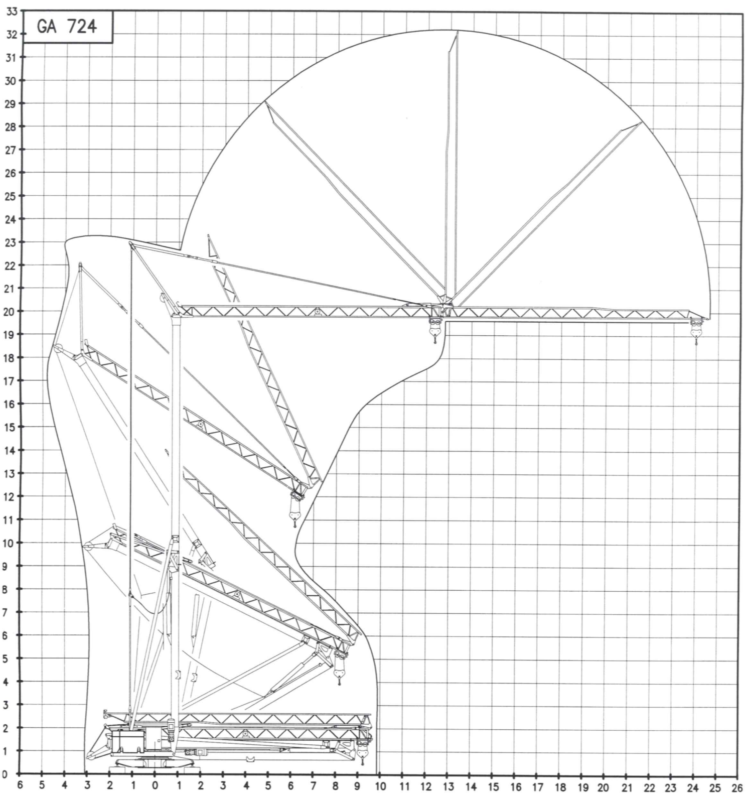
GRU IN TRASPORTO CON ZAVORRA DI MONTAGGIO
