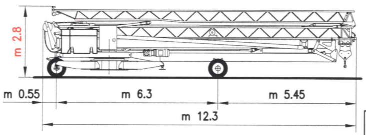
GRU IN TRASPORTO CON ZAVORRA DI MONTAGGIO
