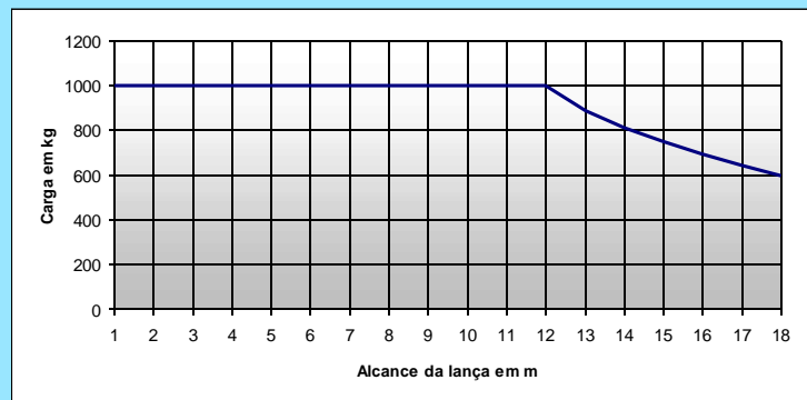
DIAGRAMA DE CARGAS / Load Diagram / Diagrama de Cargas
